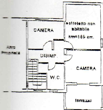
PIANO PRIMO H= 270 cm.
